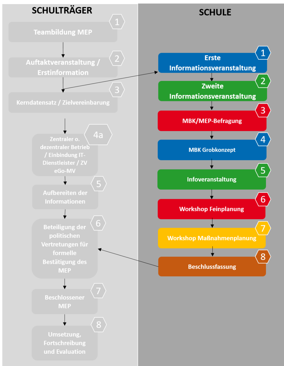
Abbildung 8: MBK Erstellungsprozess
