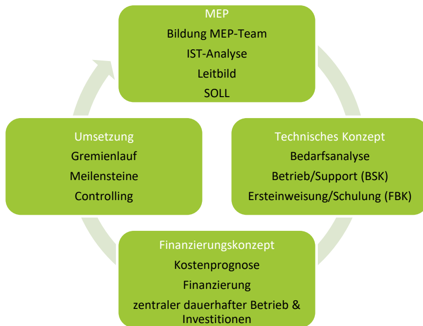
Abbildung 18: Prozess MEP
